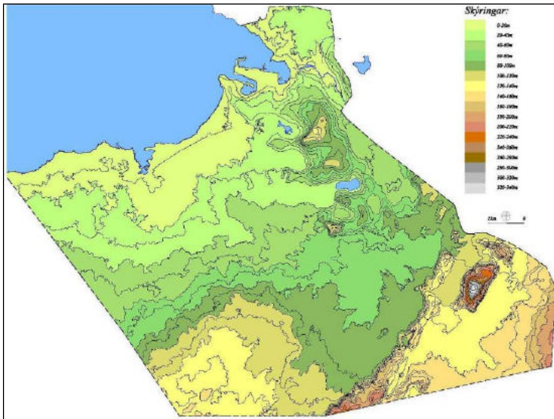
Landslag og hæðarlínufletir í landi Hafnarfjarðar
